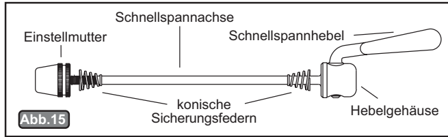
Abb. 15 Aufbau des Schnellspanners.
