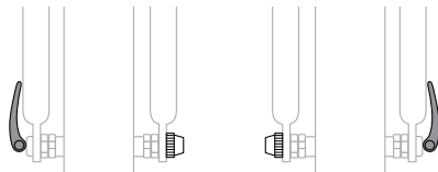
Rueda reorientada con la palanca de desbloqueo rápido en el lado opuesto
