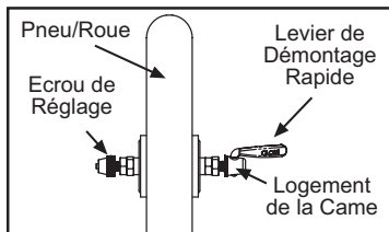
Fig. 7 Anatomie du Dispositif de Démontage Rapide de la Roue Avant
