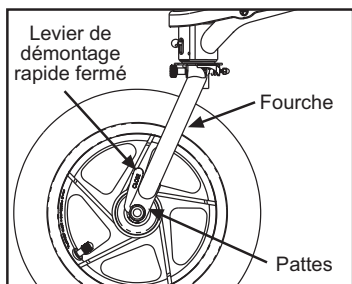
Fig. 9 Démontage rapide en position fermée, parallèle à la patte de la fourche.
