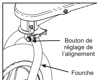
Fig. 13 Réglage de l'alignement.
