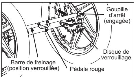
Fig. 14 Frein de stationnement – position fermée.
