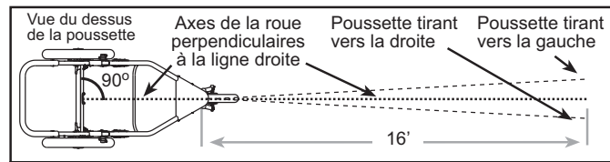
Fig. 12 Test de roulement de la poussette.
