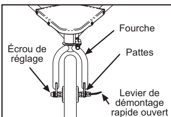
Fig. 8 Serrez l'écrou de réglage avec le levier de démontage rapide ouvert.
