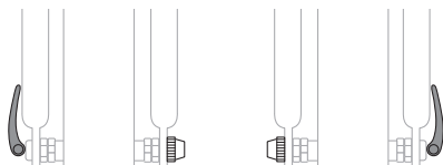
Rueda reorientada con la palanca de desbloqueo rápido en el lado opuesto
